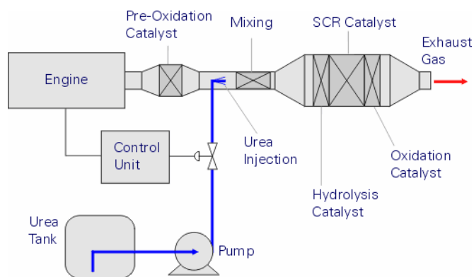
Figur 2. Princippet i et SCR-system (tv) og eksempel på et komplet system.
