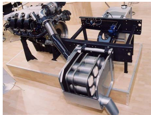
Figur 2. Princippet i et SCR-system (tv) og eksempel på et komplet system.
