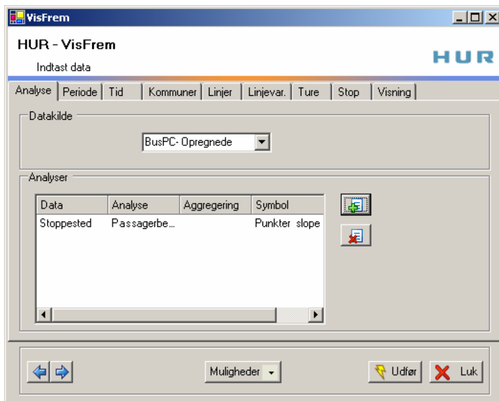
Figur 1: VisFrem brugergrænseflade
