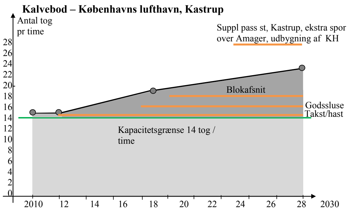
Figur 4. Lufthavnsbanen, aktuel kapacitet og forventet efterspørgselsudvikling, effekt af foreslåede tiltag
