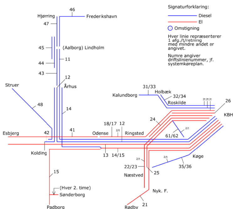
Figur 1. Driftslinjerne i Trafikstyrelsens systemkøreplan
